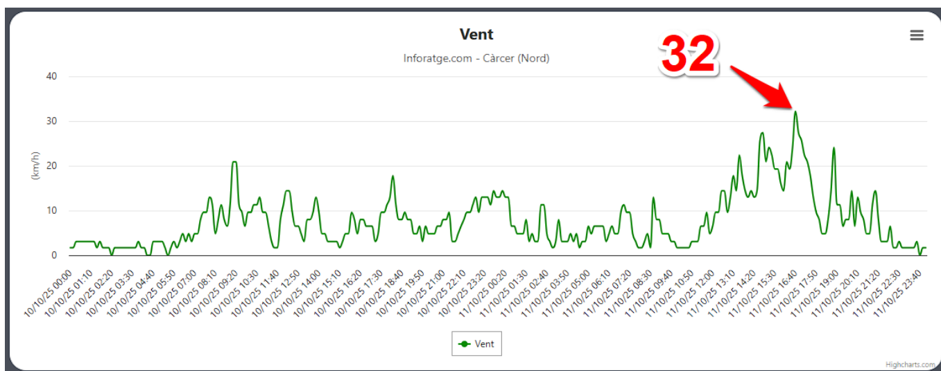
Ráfagas de viento registradas en CÀRCER (Nord) el 10 y 11/10/2025 (en km/h) https://inforatge.com/meteo-carcer
